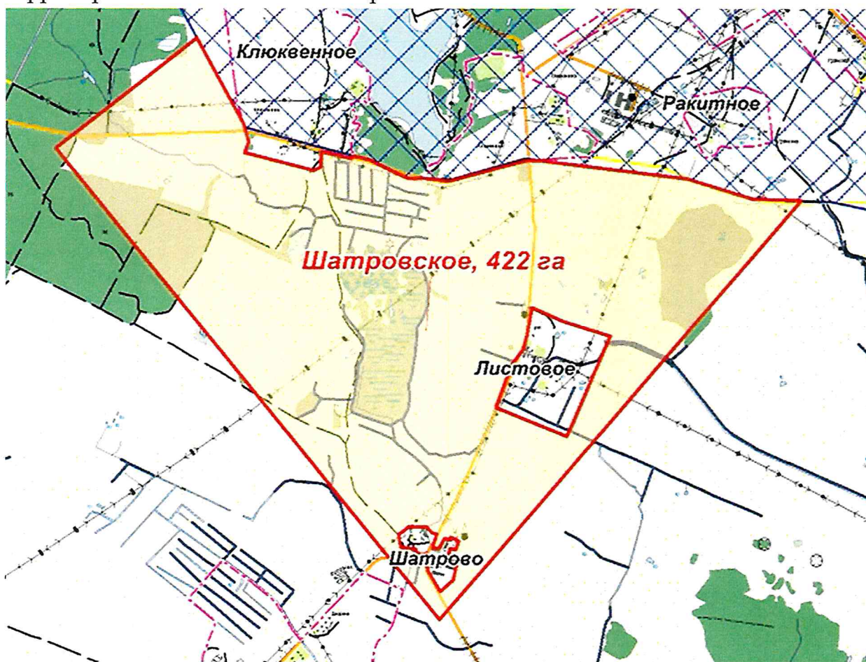
Рис. 1. Карта-схема расположения ГПЗ «Шатровское»
